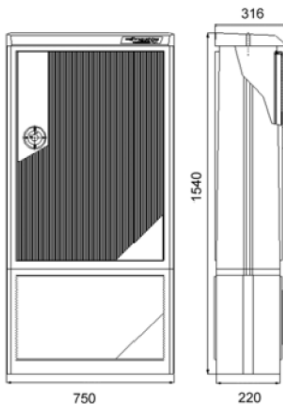
Figura 1 - Schema costruttivo dell'armadio
