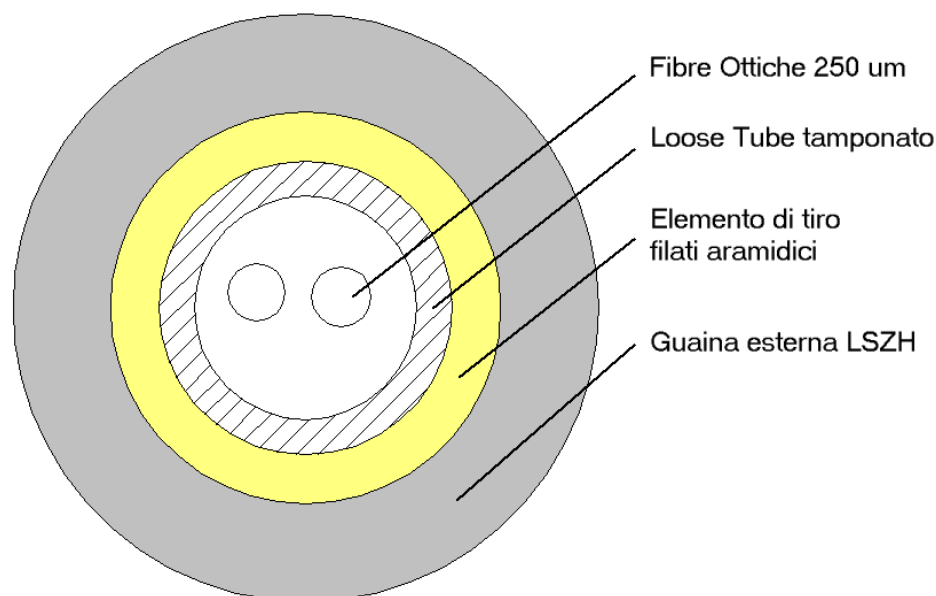
Figura 1 – Cavo fibre ottiche 2FO
